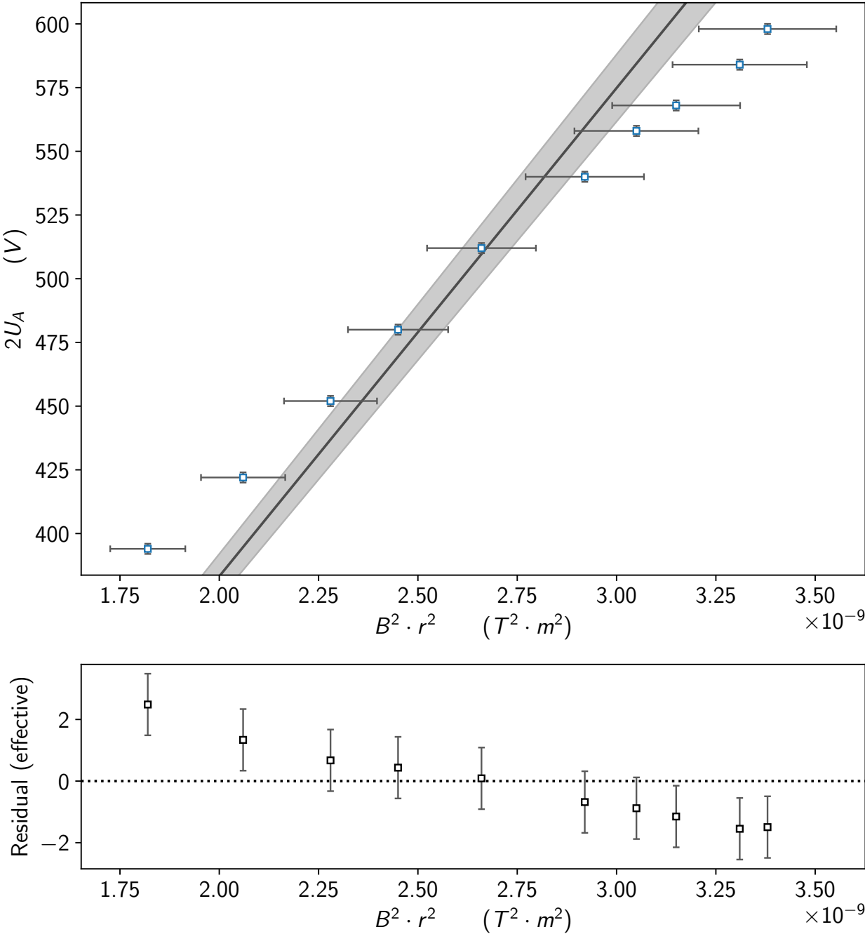
Ajuste lineal con b=0 para trayectoria circular de radio r= 4 cm
