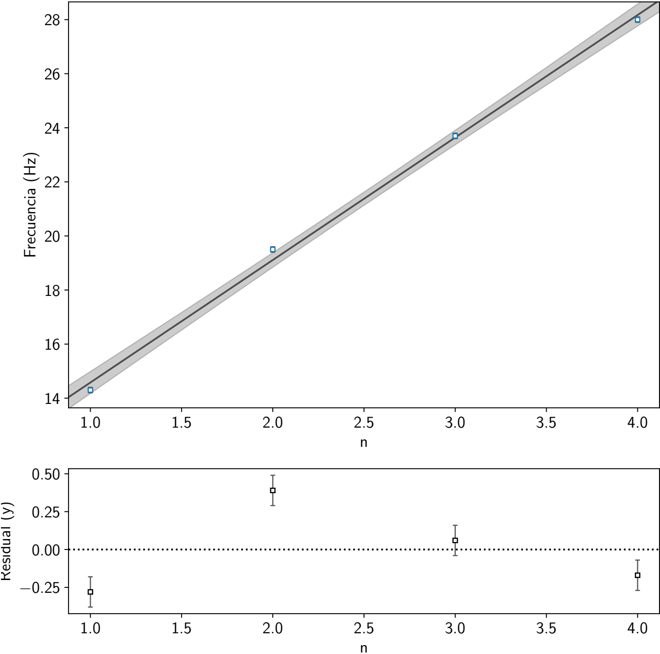
Frecuencia frente a numero armonico
