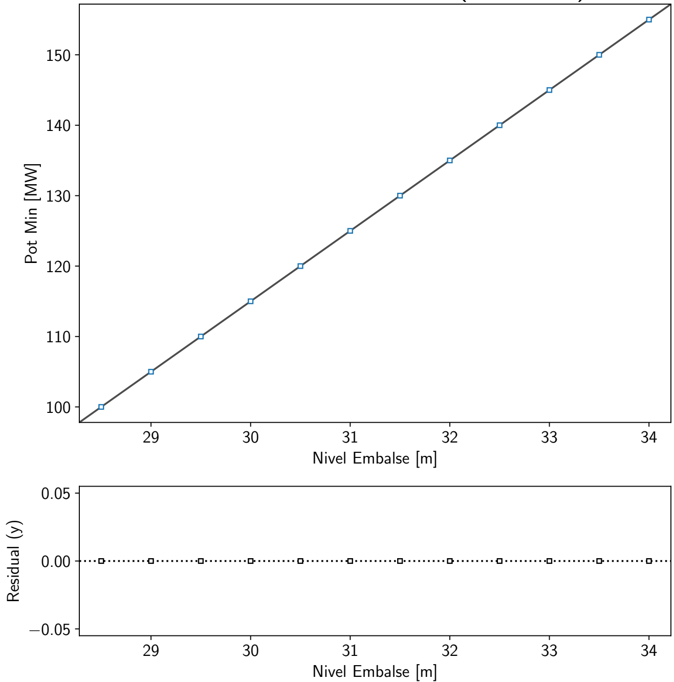
Pot min vs Embalse - Tramo 2 (22 - 23,5 m)
