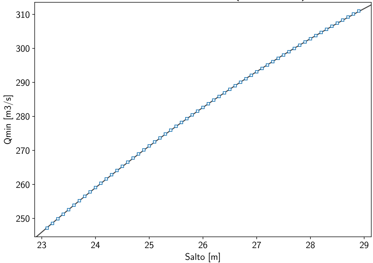
Qmin vs Salto - Tramo 4 (23 - 28,9 m)
