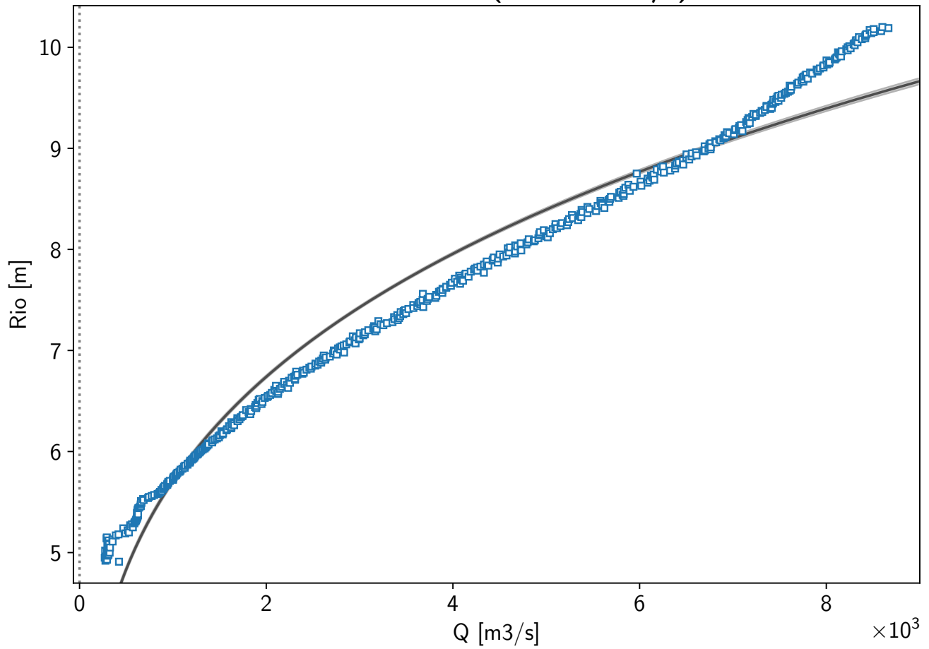
Rio vs Caudal (0 - 8600m3/s)
