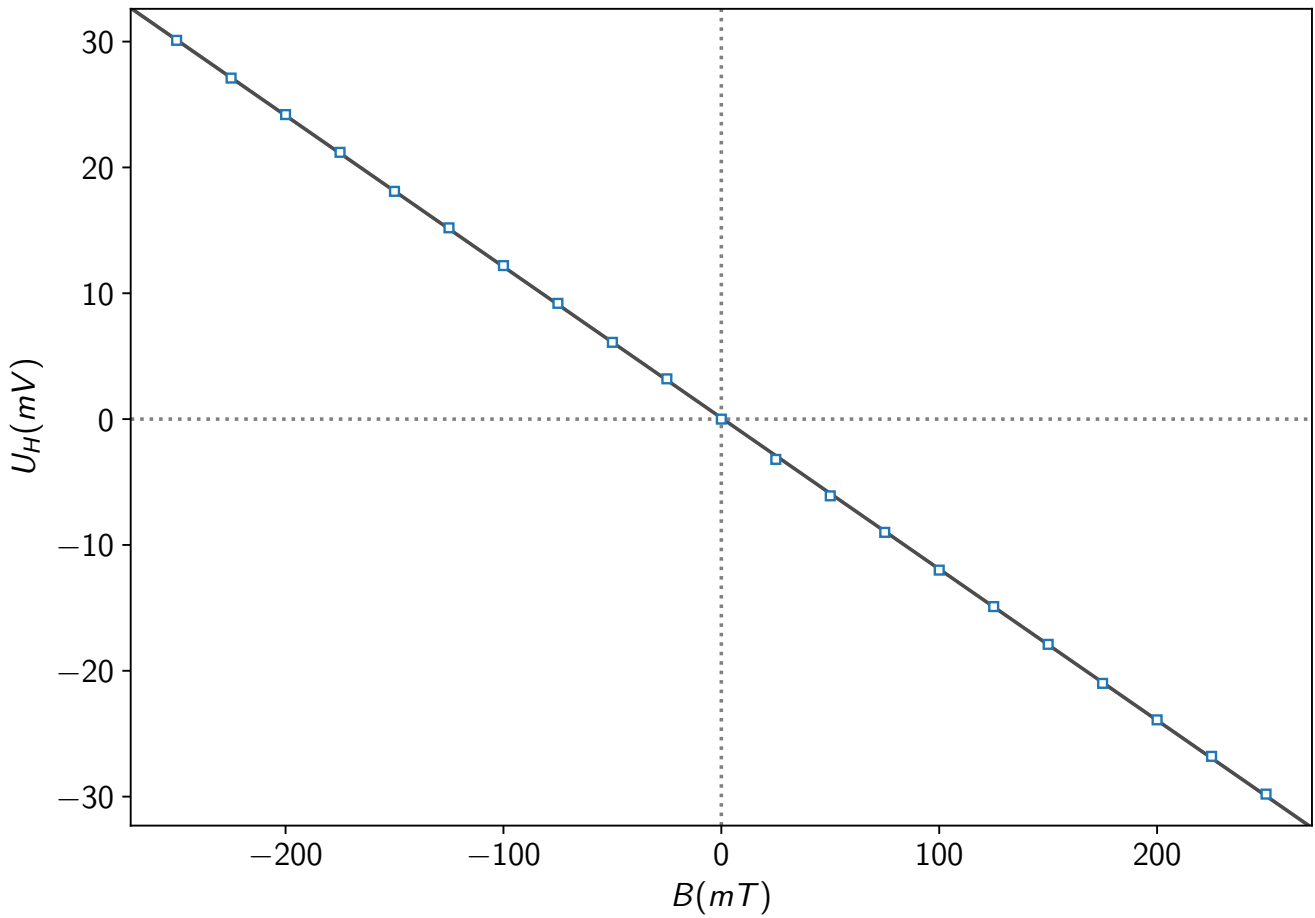
Germanio n, I = 15\text{mA}
